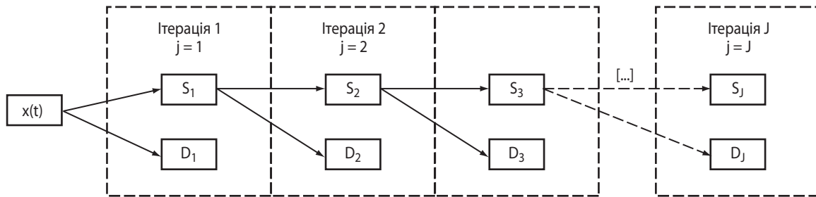
Рис. 2. Алгоритм розкладання сигналу з використанням вейвлет-функцій
