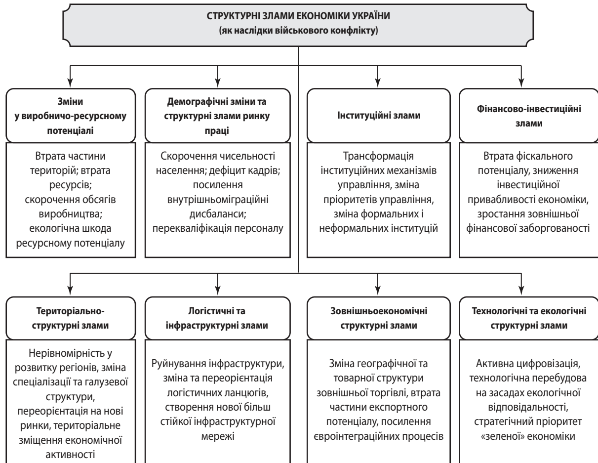
Рис. 2. Структурні зміни у національній економіці України
