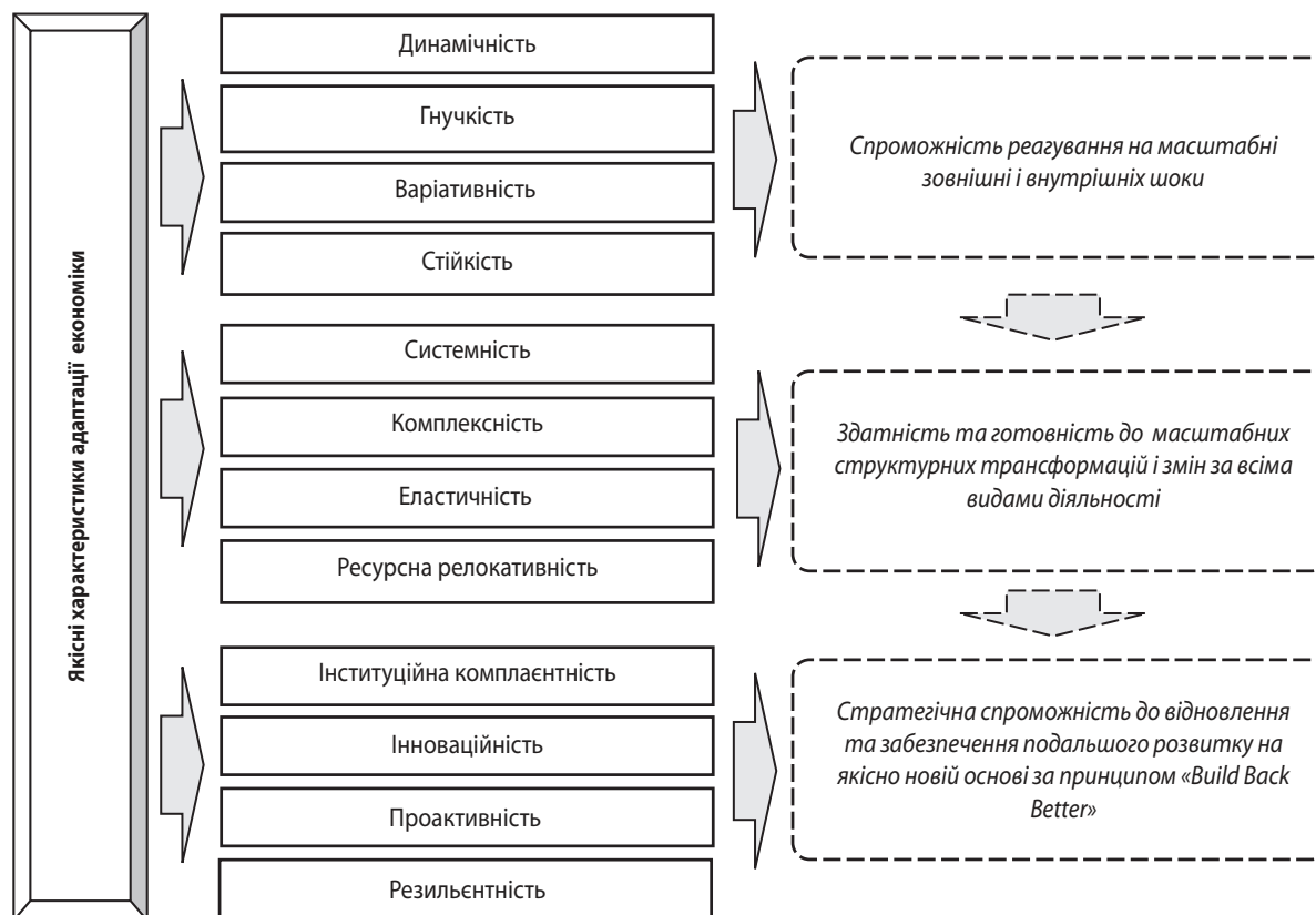
Рис. 1. Якісні характеристики адаптації економіки країни до структурних змін та зовнішніх і внутрішніх шоків
